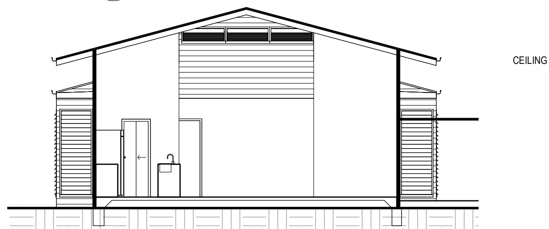
3 MAIN SECTION 1 : 100
