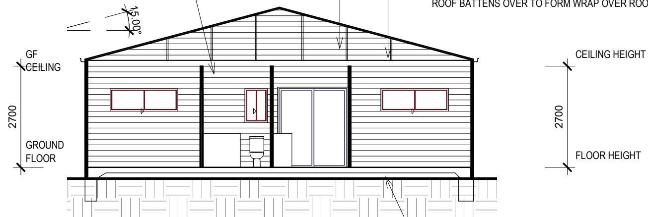
1 BEDROOM SECTION 1 : 100
