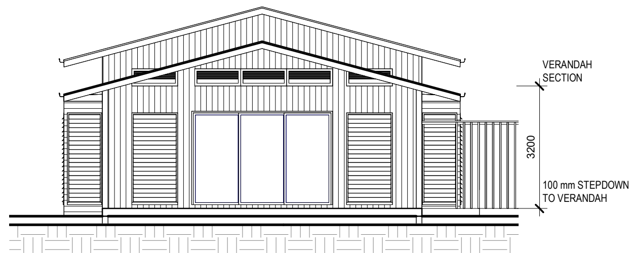
2 VERANDAH SECTION 1 : 100
